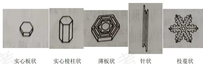
雪晶形态图
